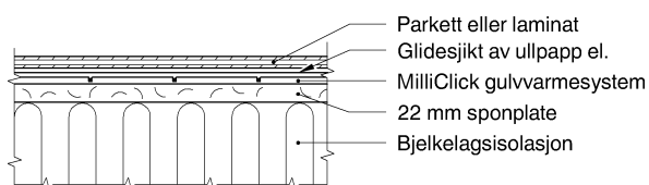
Fig. 3. Silencio EL gulvvarmesystem lagt direkte på 22 mm sponplater i mellombjelkelag.
