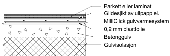
Fig. 4. Silencio EL plater lagt direkte på avrettet, isolert betonggulv (f.eks. gulv på grunnen).
