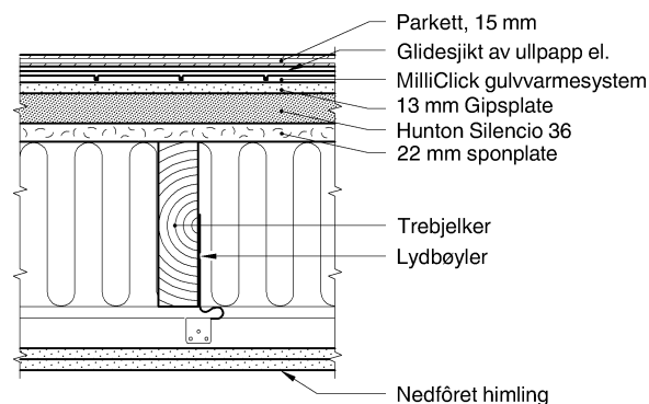
Fig. 5. Gulv med Silencio EL over Silencio Hunton 36 på etasjeskiller av trebjelkelag med lydhimling.
